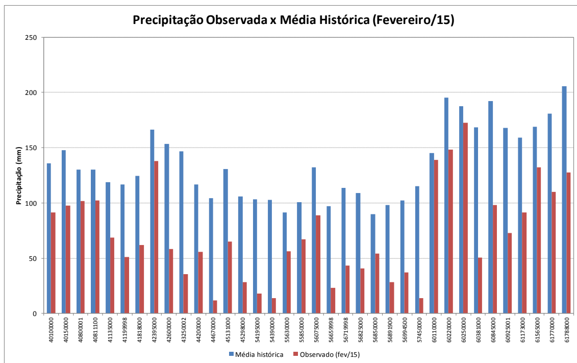
Figura 6 – Comparação entre a precipitação acumulada até 25 de fevereiro de 2015 e a média histórica de fevereiro de 1998 a 2014 por estação
