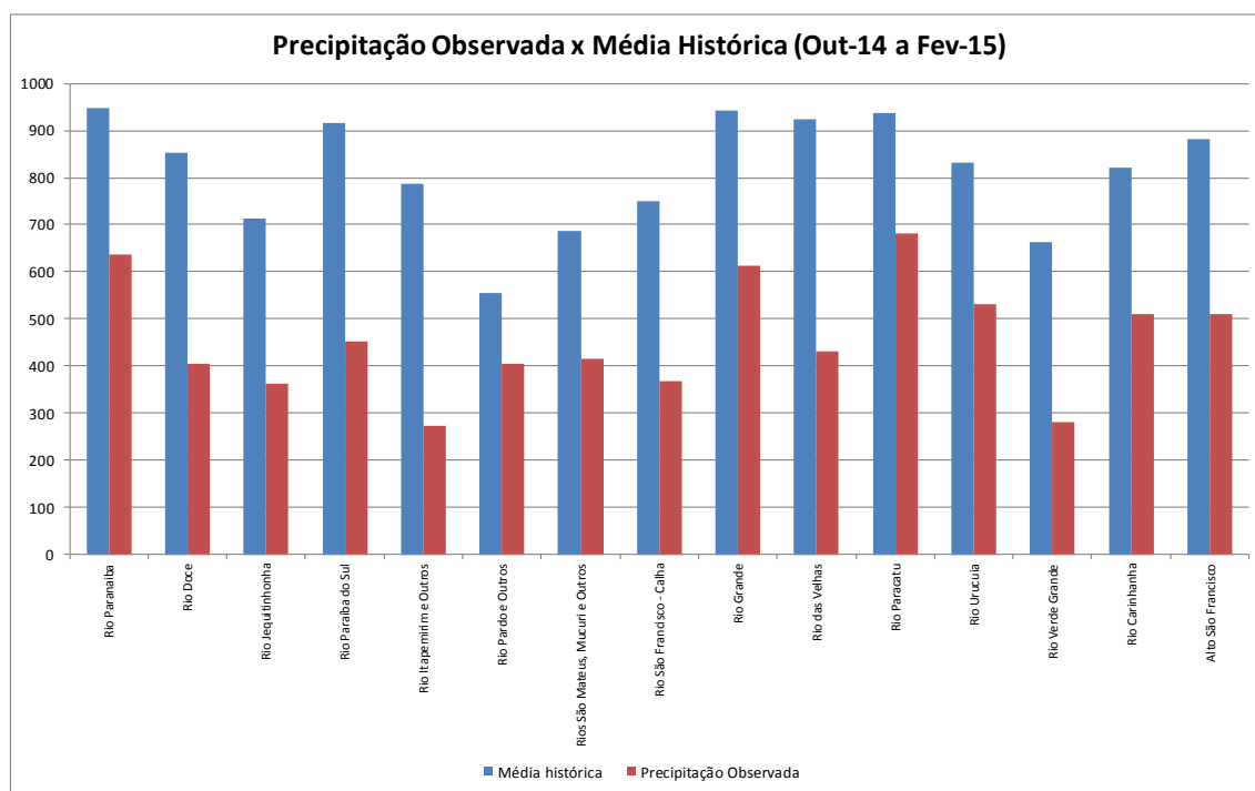
Figura 4 – Comparação entre a precipitação média acumulada de outubro a fevereiro e a observada no período de outubro de 2014 a 25 de fevereiro de 2015.
