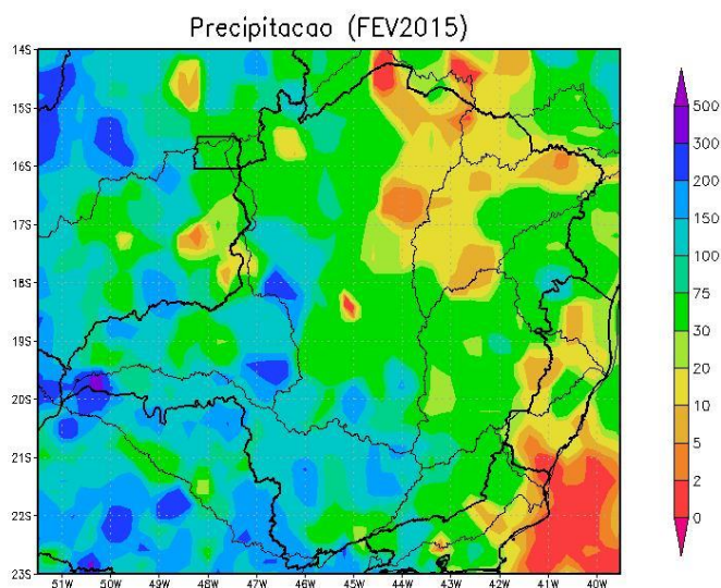
Figura 2 - Precipitação acumulada até 25 de fevereiro de 2015.
